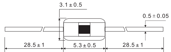
Dimensions(mm)尺寸
